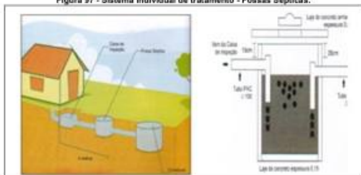
Figura 97 - Sistema individual de tratamento - Fossas Sépticas.
