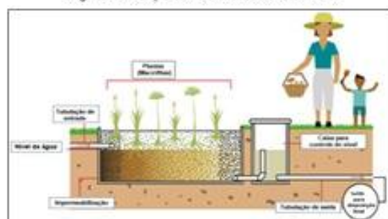
Figura 103 - Esquema de Zona de Raízes ou SAC.
