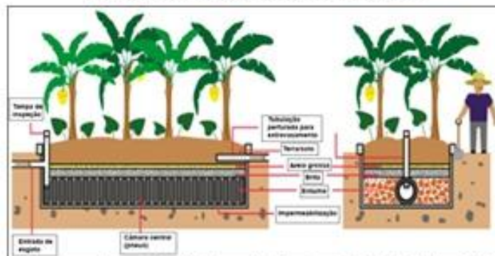
Figura 107 - Esquema de bacia de evapotranspiração - BET.
