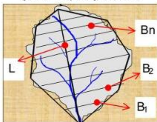
Figura 81 - Determinação da largura média da bacia.
