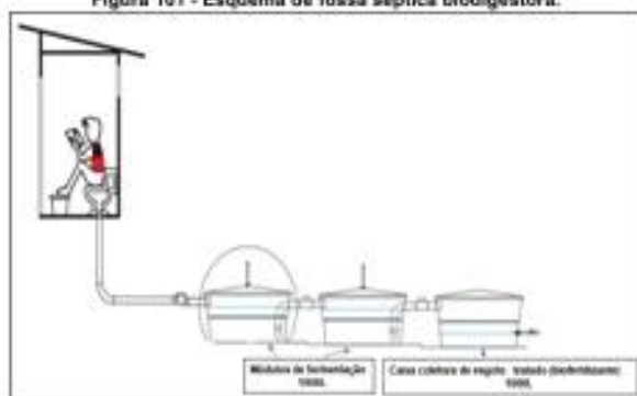
Figura 101 - Esquema de fossa séptica biodigestora.
