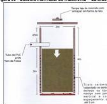
Figura 99 - Sistema individual de tratamento - Sumidouros.
