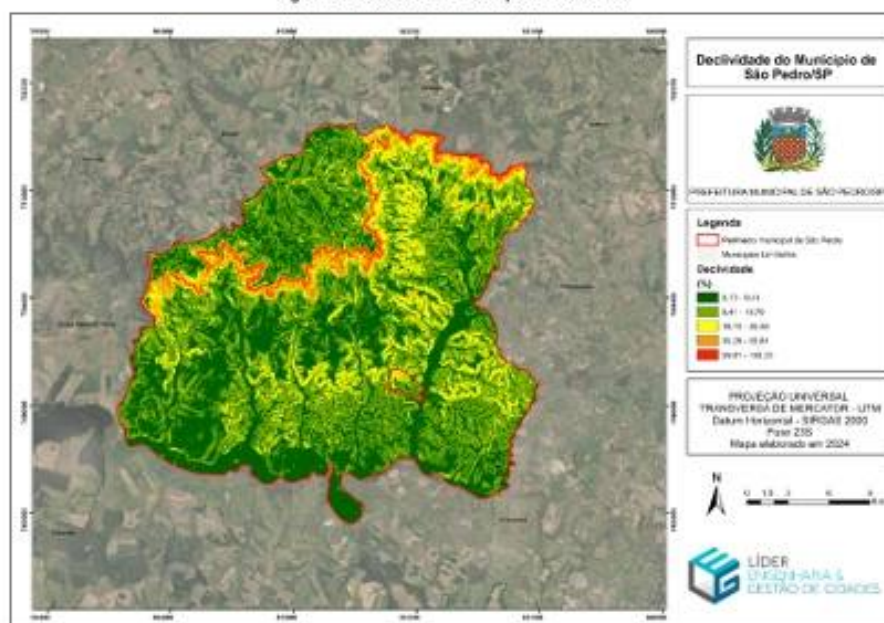
Figura 9 - Declividade do município de São Pedro.
