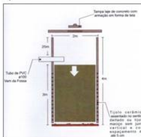
Figura 54 – Sistema individual de tratamento – Sumidouro.
