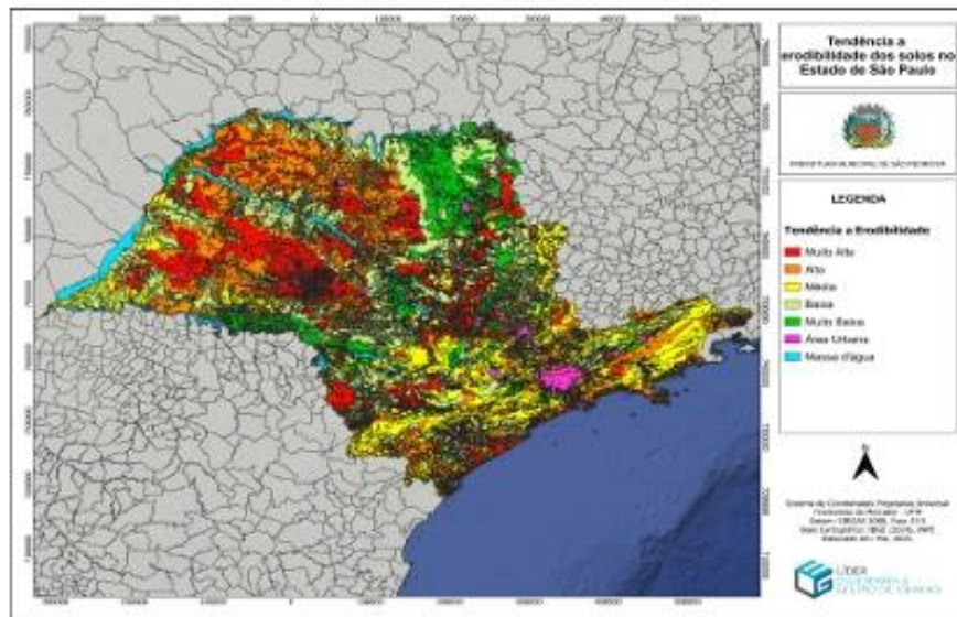
Figura 87 - Erodibilidade dos solos no Estado de São Paulo.
