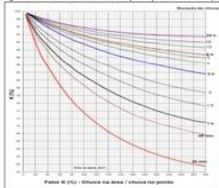
Figura 82 – Coeficiente de distribuição espacial da chuva (K).
