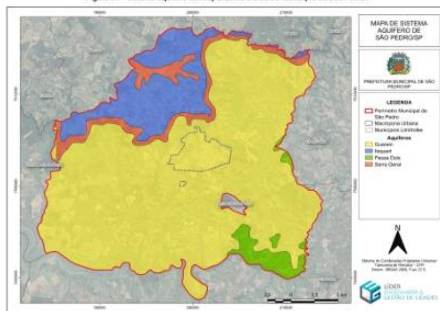
Figura 34 – Sistema aquífero correspondente à área do Município de São Pedro.
