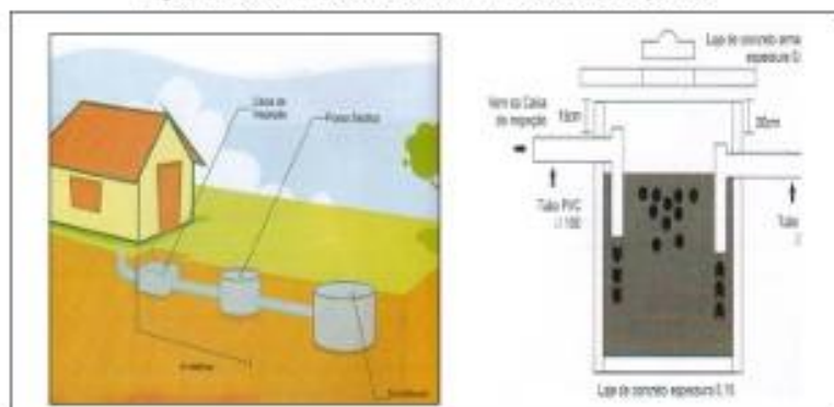
Figura 52 - Sistema Individual de Tratamento – Fossas Sépticas.
